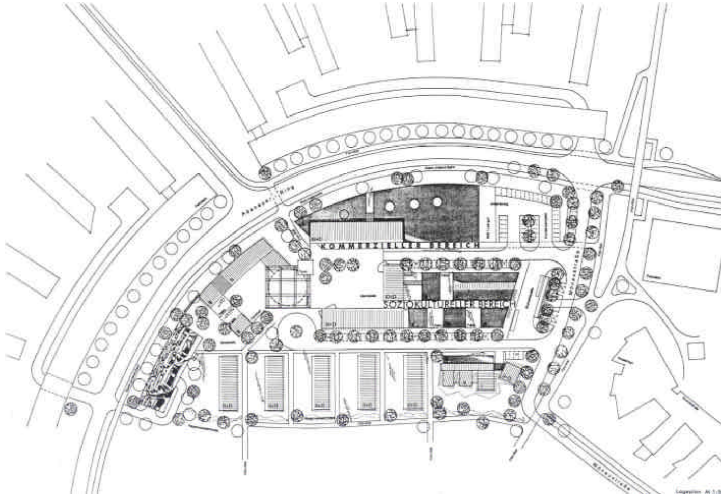
Lageplan
