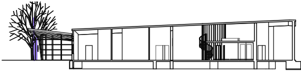
Schnitt 1-1
