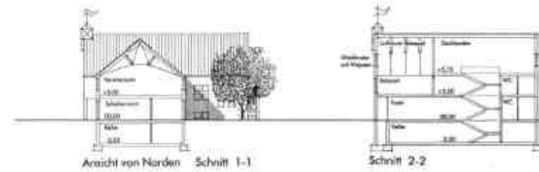
Ansicht von Norden Schnitt 1-1
