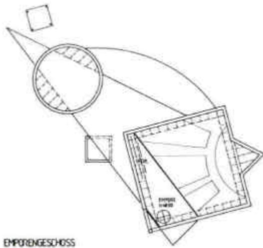
EMPORENGESCHOSS
